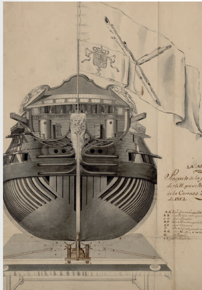
Dibujo de la proa del navio «La África».
